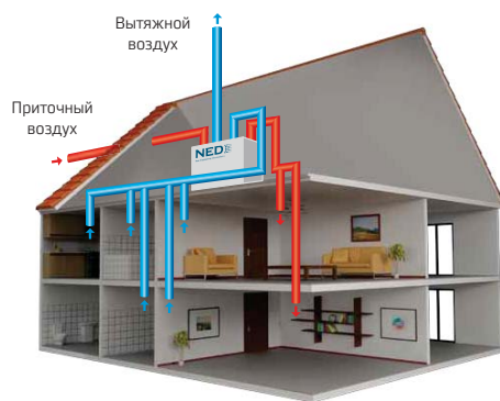
СХЕМА РАБОТЫ УСТАНОВКИ MININED В ЖИЛОМ ПОМЕЩЕНИИ
