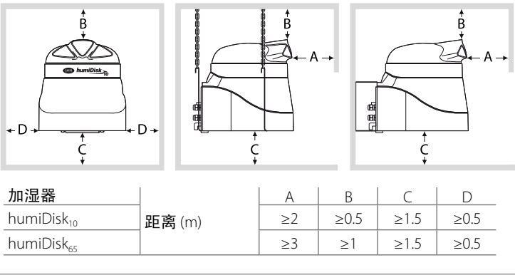
湿度调节器
