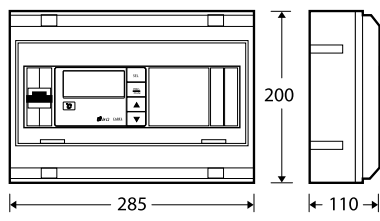
控制板
